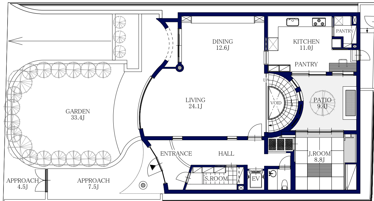
1階平面図
