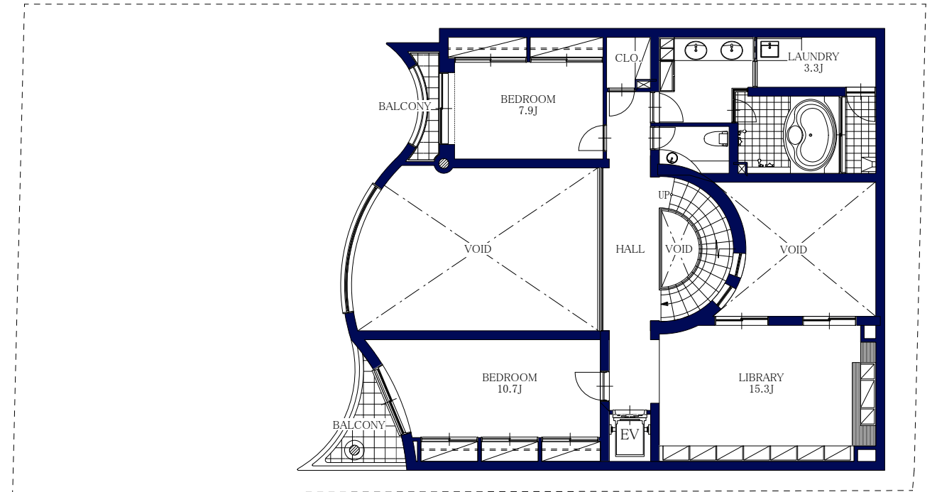
2階平面図
