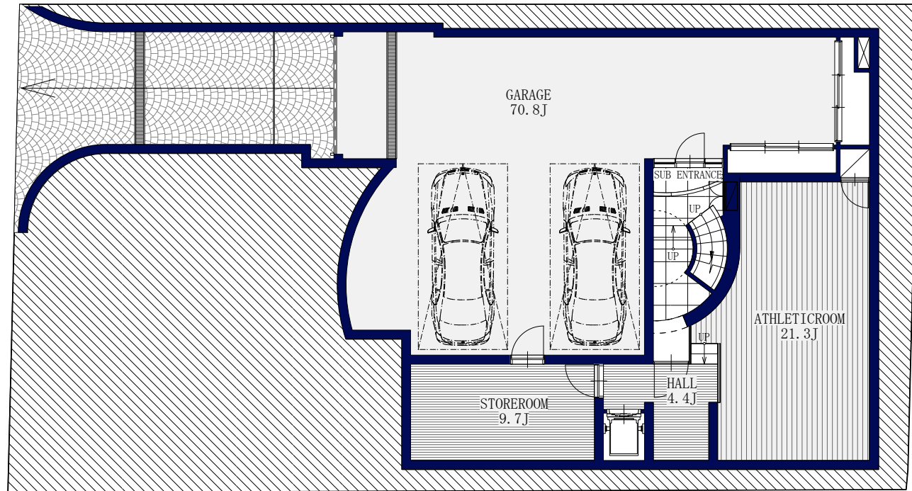
地階平面図
